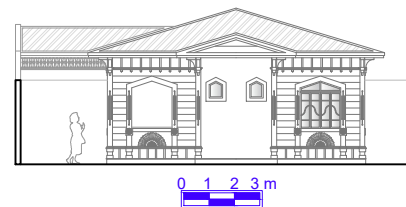
Elevação 03
