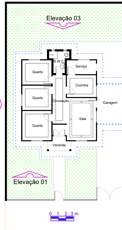
Planta
