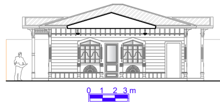
Elevação 02
